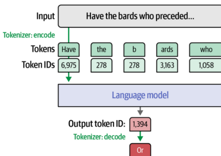
Figura 2.15: Tokenizador: decodificación
