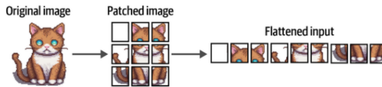
Figura 2.28: Tokenización de una imagen como entrada
