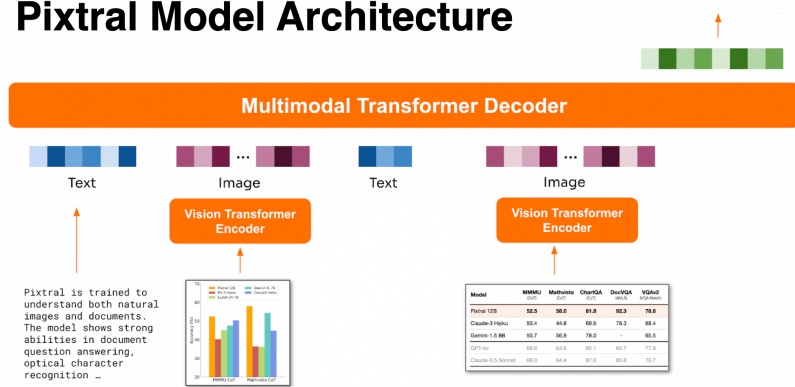
Figura 4.5: Arquitectura de Pixtral-12b
