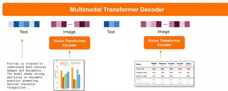
Figura 4.5: Arquitectura de Pixtral-12b
