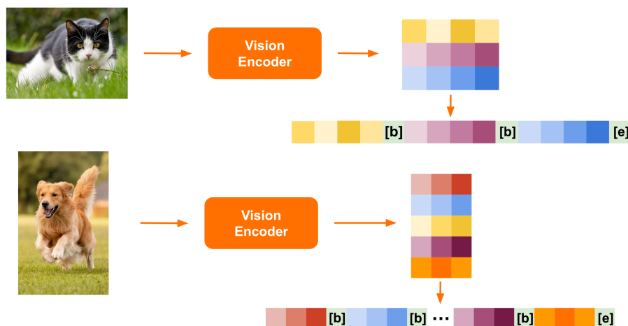
Figura 4.5: Funcionamiento del codificador de visión de Pixtral-12b
