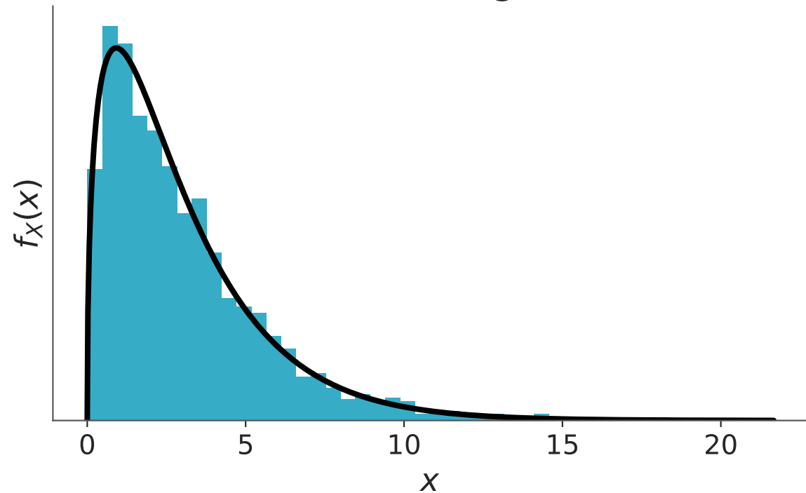
Gamma(mu=3, sigma=2.5)
