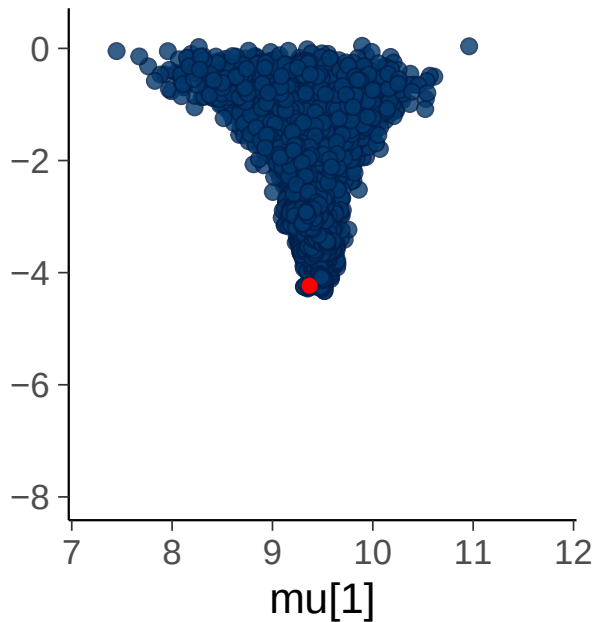
CP + adapt_delta=0.999
