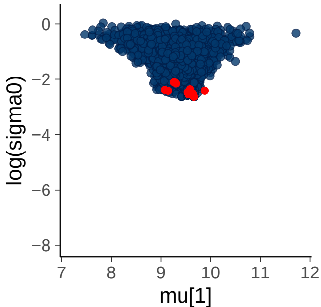
CP + adapt_delta=0.8
