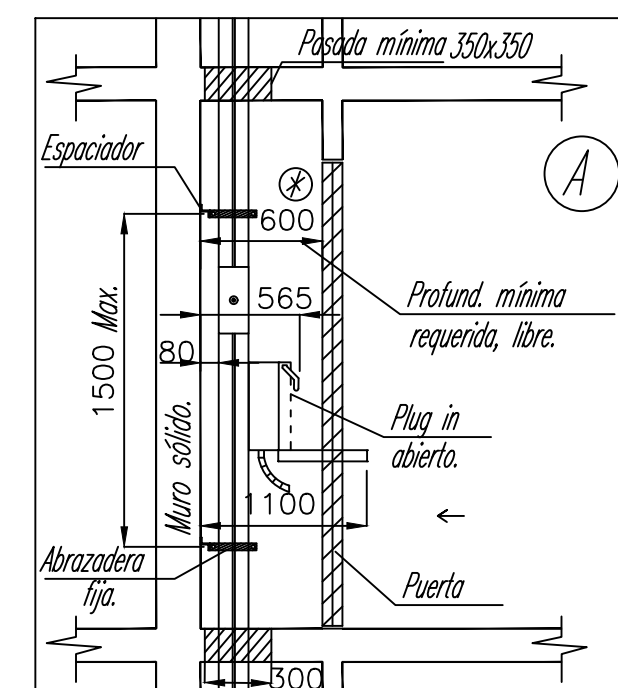
Detalle manto arribo XCM 400-1000A.
