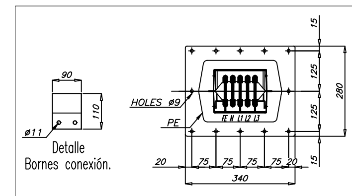
Detalle manto arribo XCM 400-1000A.
