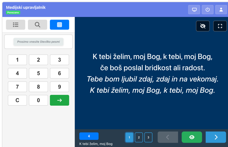
Slika 2: Glavna navigacija (gumbi na vrhu) in pogled projekcije
