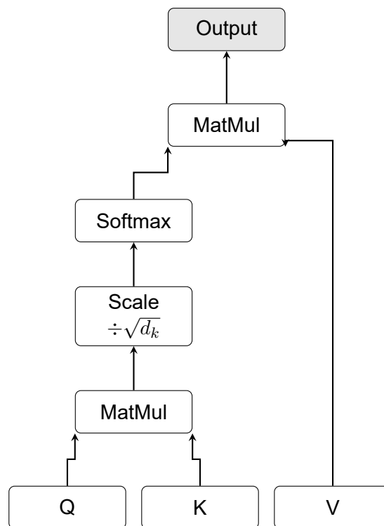
איור 3.1: ארכיטקטורת Scaled Dot-Product Attention.
