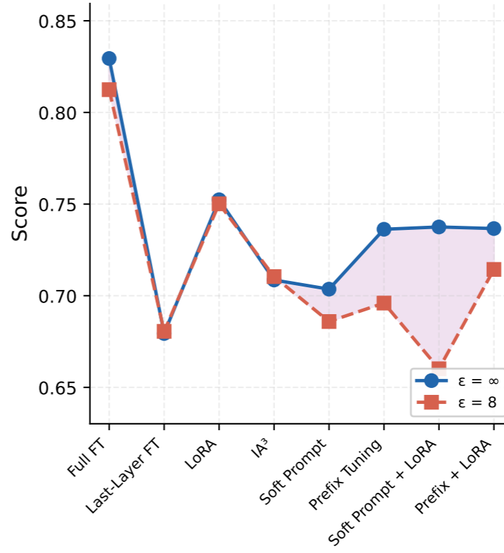
QQP
