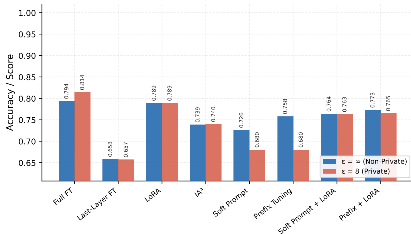
QQP
