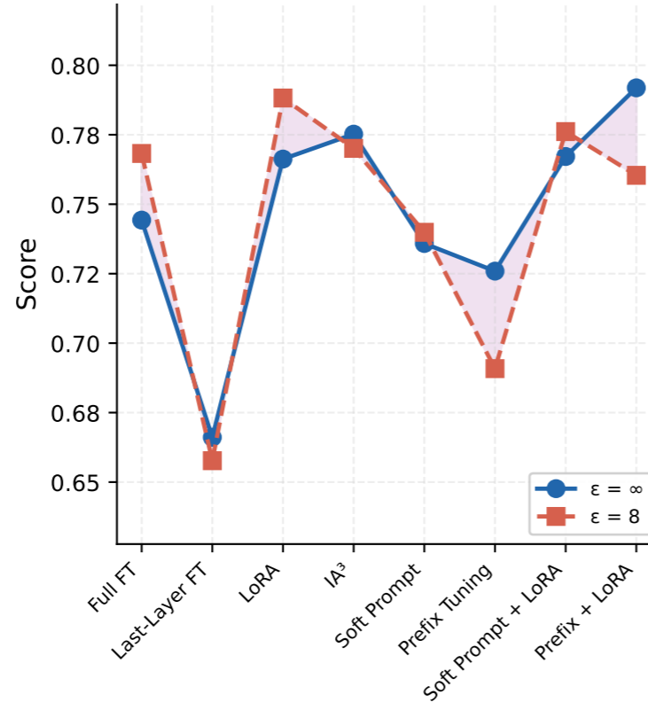
QNLI
