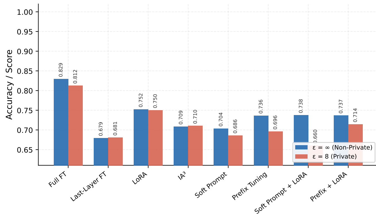
QQP
