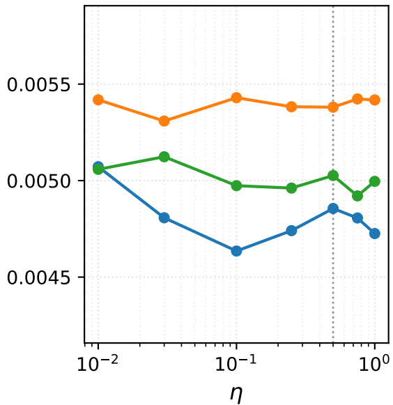
Matrix RIAE
