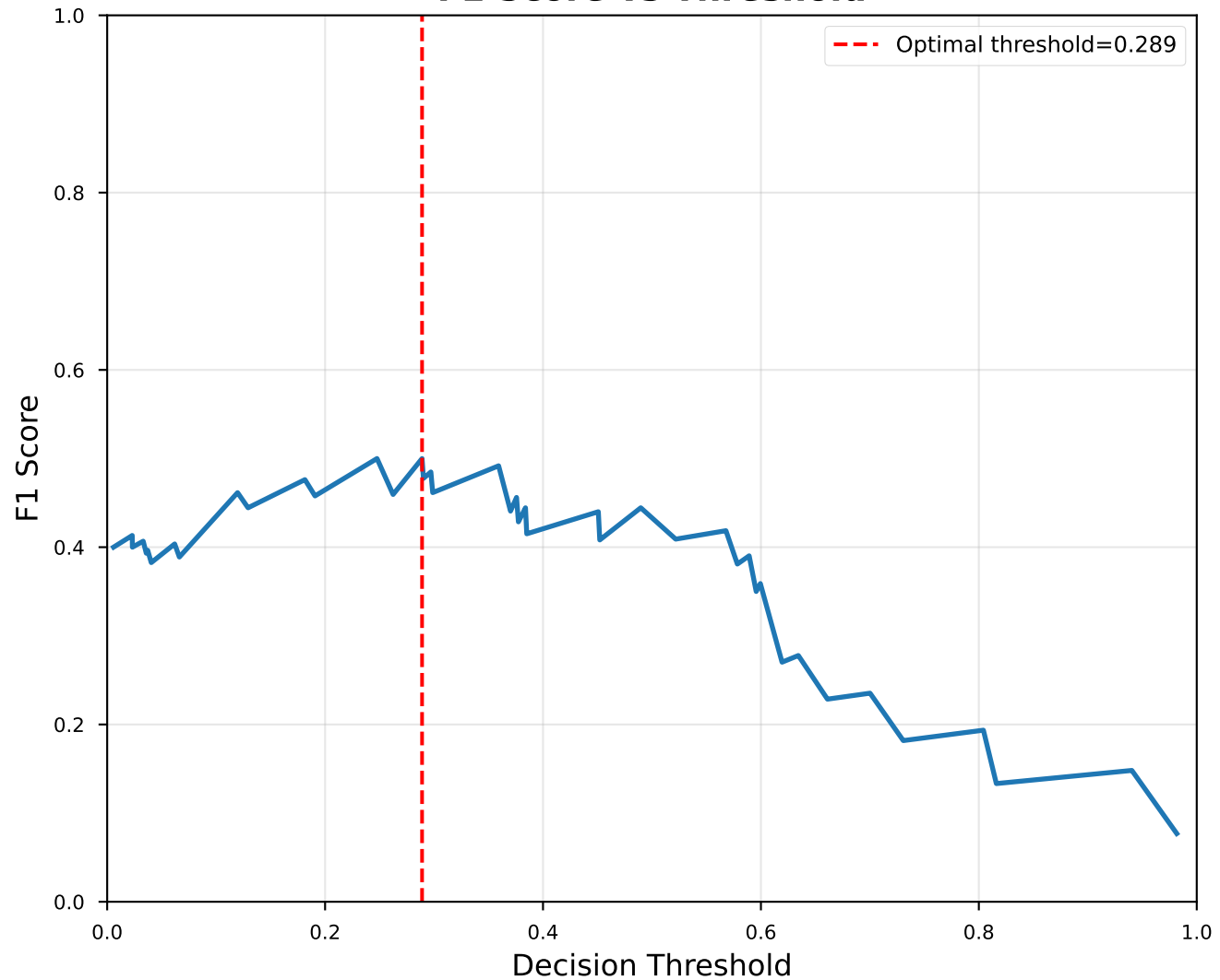
F1 Score vs Threshold
