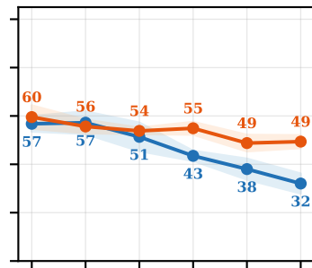
OpenVLA
