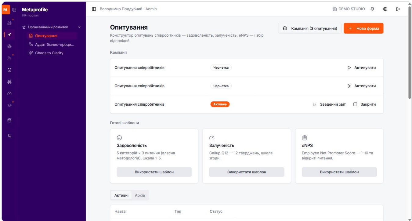
Екран «Опитування»: угорі кампанії, нижче — готові шаблони (Задоволеність, Залученість, eNPS)
