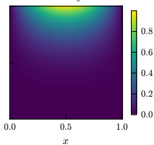
LiL u_y
