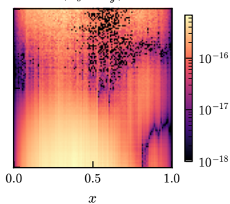
|u_y - u_y^*|
