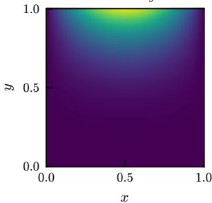
Exact u_y
