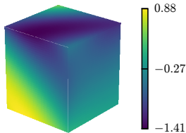
LiL-Q v
