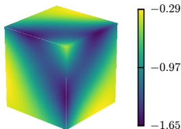
LiL-Q p
