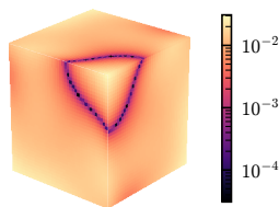
|p - p^*|
