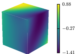
LiL-Q w
