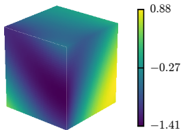
Exact w
