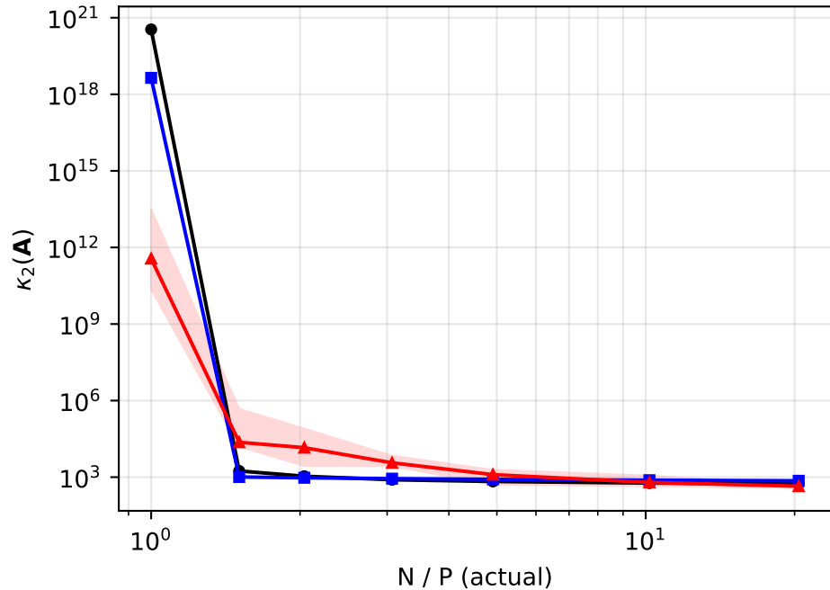
kovasznay, P = 300
