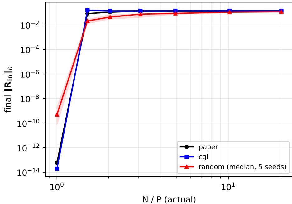
kovasznay, P = 300
