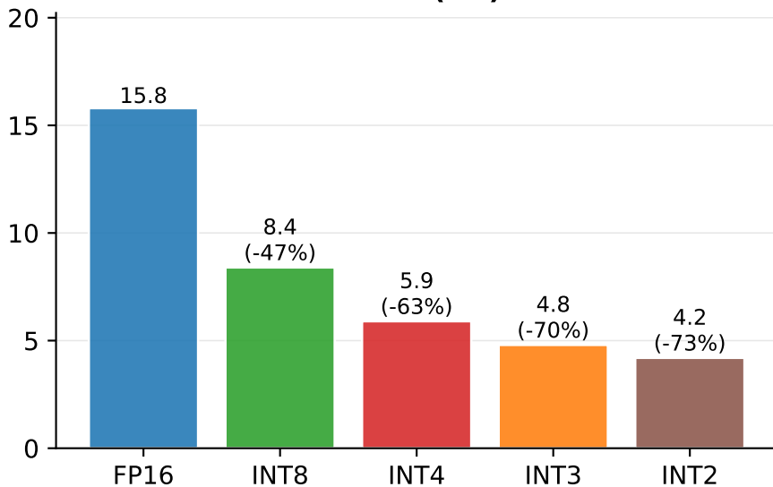
Latency (ms/token)
