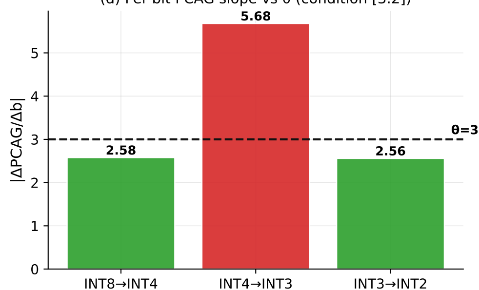
(d) Per-bit PCAG slope vs \theta (condition [3.2])
