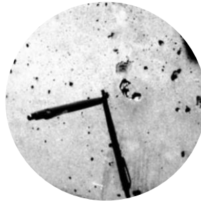
Bugholes: Cavidades irregulares que no exceden los 15 mm de diámetro.
