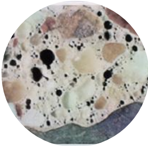
Vacío de aire
