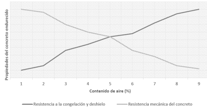
Efecto del contenido de aire del concreto en sus propiedades en estado endurecido
