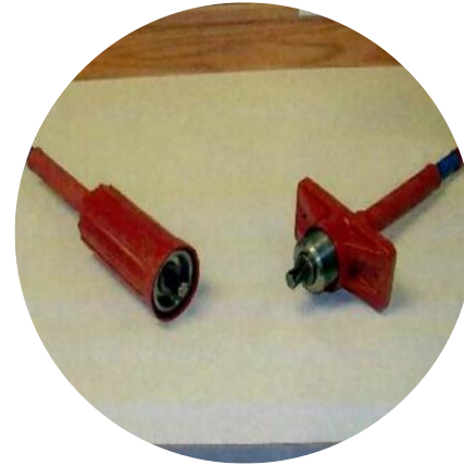
Anclaje intermedio, Anclajes intermediantes/ Intermediate anchorage
