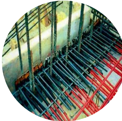
Refuerzo de rotur/Bursting steel
