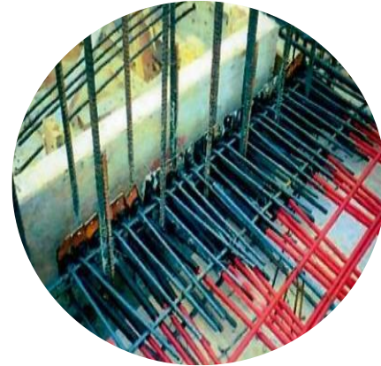
Molde de borde/Edge form
