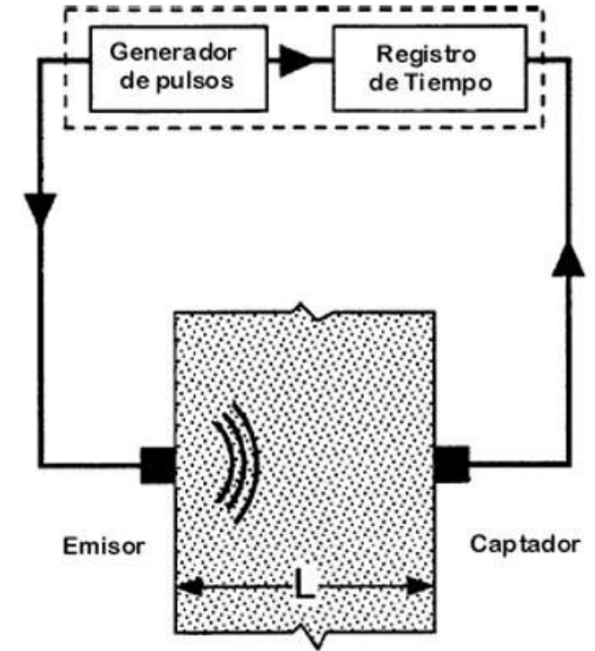
Esquema del aparato para medir la velocidad del pulso ultrasónico.
