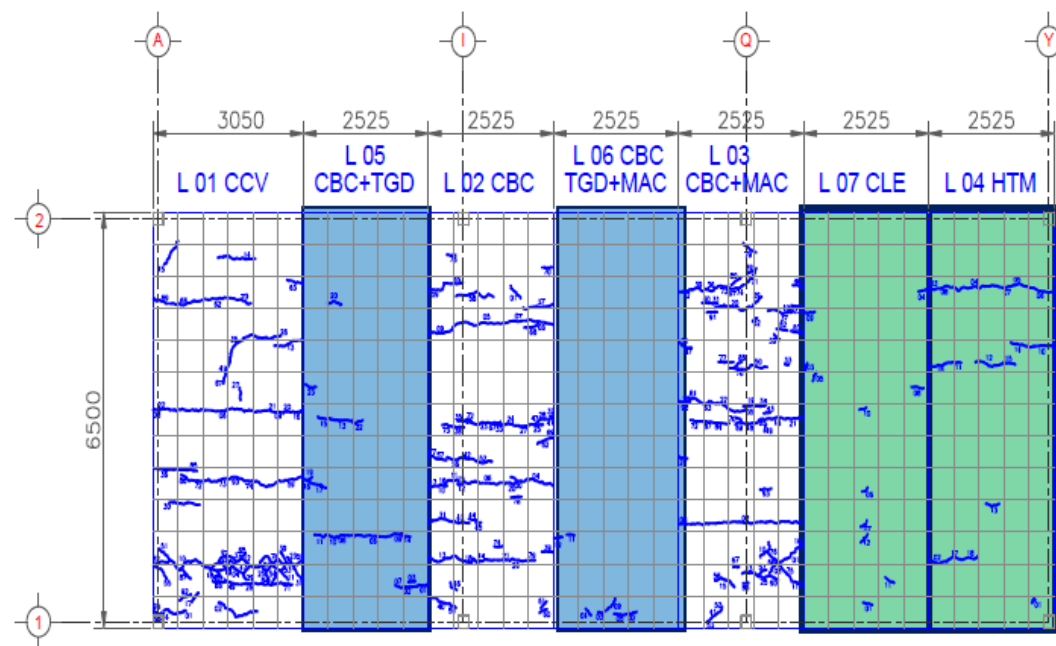
Agrietamiento por contracción a 90 días
