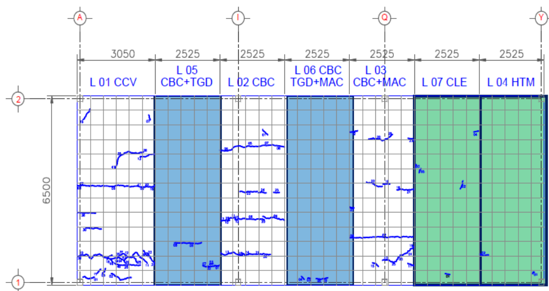
Agrietamiento por contracción a 28 días
