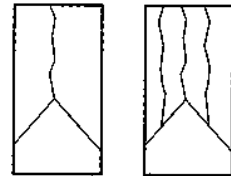
Tipo 2 Conos bien formados en un extremo, fisuras verticales a través de los cabezales, pero no bien definidos en el otro extremo
