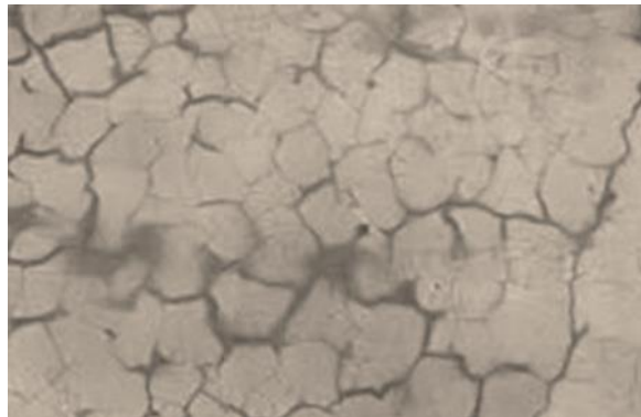
AGRIETAMIENTO POR TEMPERATURA
