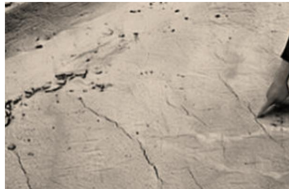
AGRIETAMIENTO POR CONTRACCIÓN PLÁSTICA
