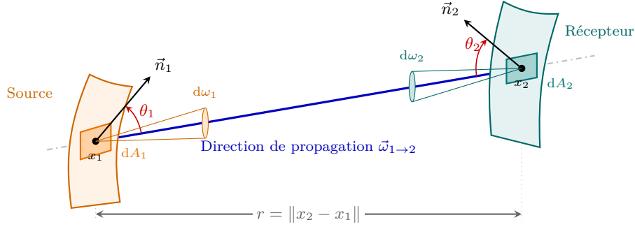
FIGURE 2.2 – Transport radiatif différentiel entre deux éléments de surface orientés dA_1 et dA_2 séparés par une distance r .
