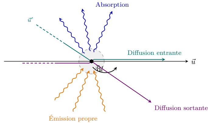
FIGURE 2.3 – Bilan des interactions locales de l'ETR en un point matériel x sur l'élément de longueur dl le long de la direction \vec{u} .
