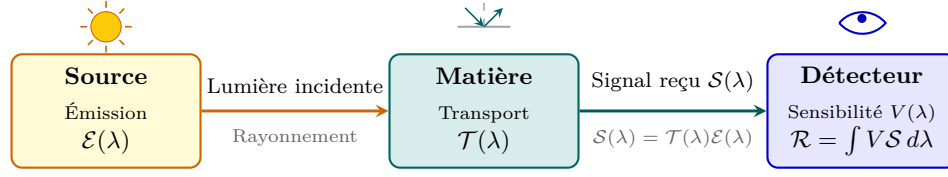
FIGURE 2.1 – Chaîne fondamentale de formation de l'image en synthèse d'images : de l'émission à la réponse du capteur.
