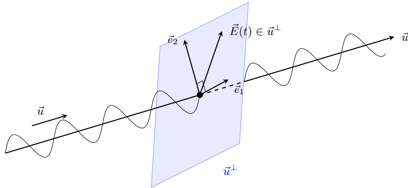
FIGURE 2.4 – Propagation libre le long de \vec{u} et confinement de l'oscillation transverse \vec{E}(t) dans le plan orthogonal \vec{u}^\perp = \text{Vect}(\vec{e}_1, \vec{e}_2) .
