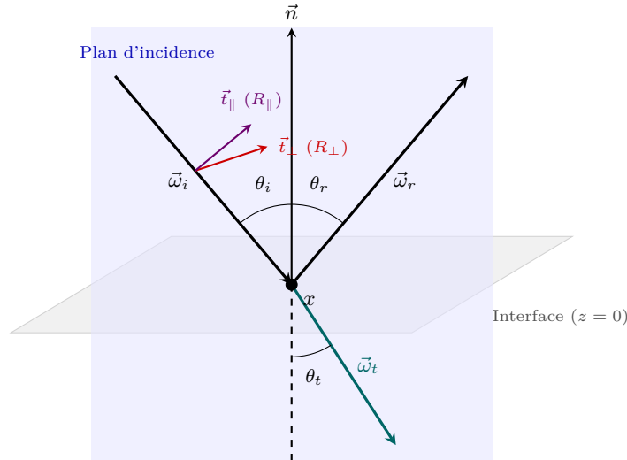
FIGURE 2.5 – Décomposition des composantes de polarisation orthogonale ( R_{\perp} ) et parallèle ( R_{\parallel} ) par rapport au plan d'incidence.
