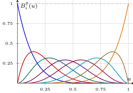
(a) Base de Bernstein de degré 7 ( B_0^7, \dots, B_7^7 )
