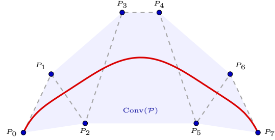
(b) Aplatissement de la courbe paramétrique
