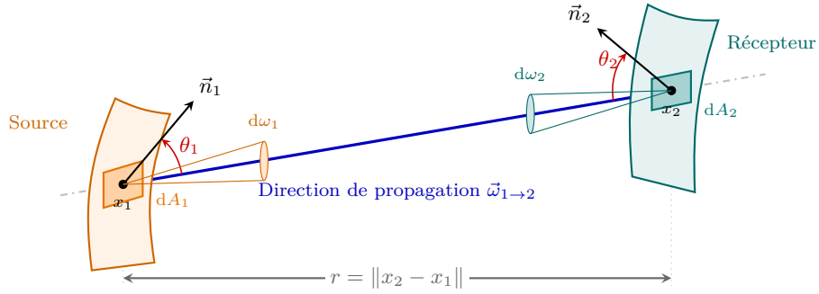
FIGURE 2.2 – Transport radiatif différentiel entre deux éléments de surface orientés dA_1 et dA_2 séparés par une distance r .
