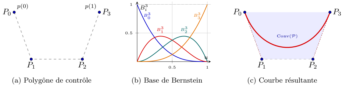
FIGURE 1.2 – Construction d'une approximation de Bézier cubique : du polygône de contrôle au tracé final borné par l'enveloppe convexe.
