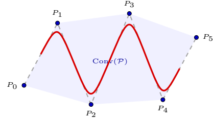
(b) Courbe lissée C^1 par morceaux
