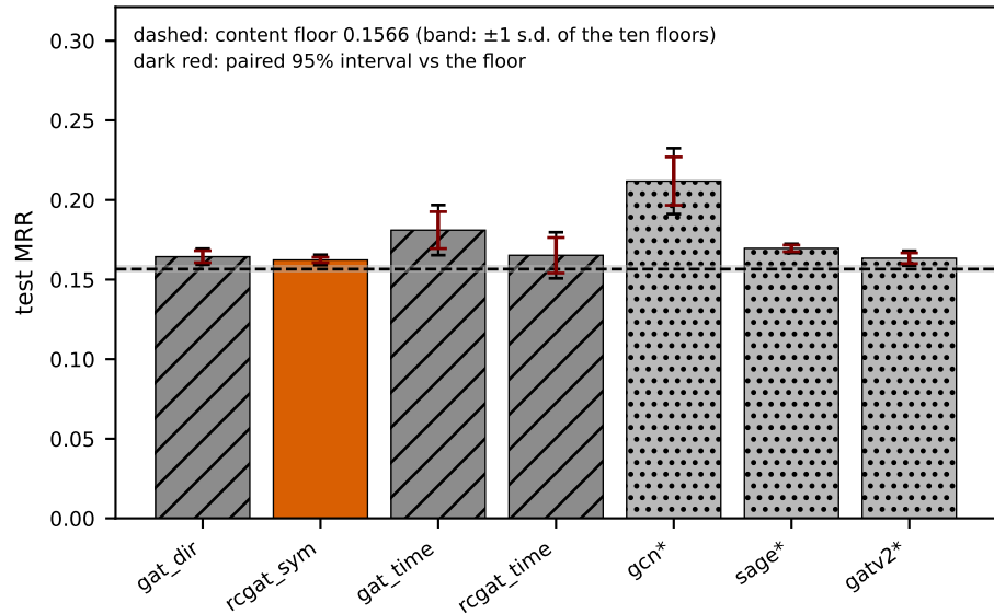
npm
