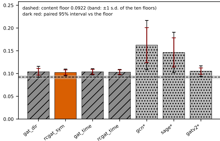
Maven
