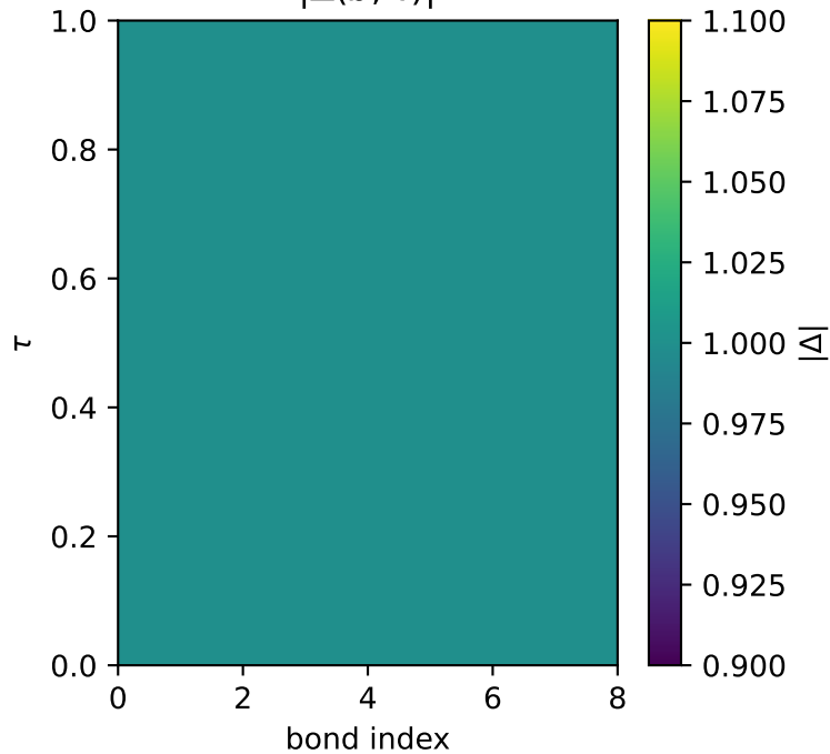
|\Delta(b, \tau)|
