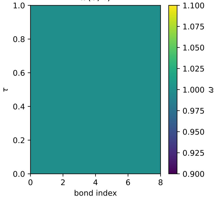
\omega(b, \tau)
