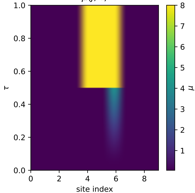
\mu(j, \tau)
