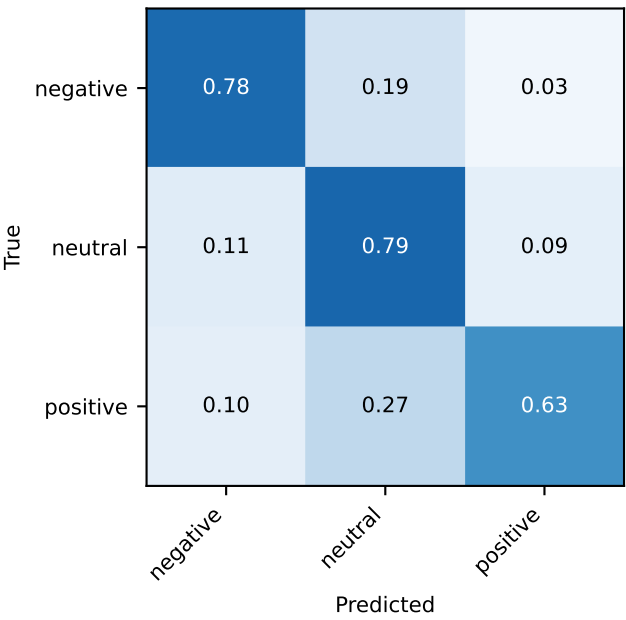
FinGPT-Llama-3-8B-LoRA
