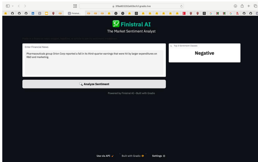
Fig. 3: Finistral-7B-LoRA GUI
