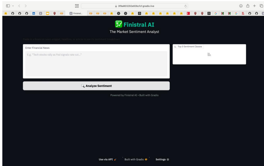
Fig. 2: Finistral-7B-LoRA GUI
