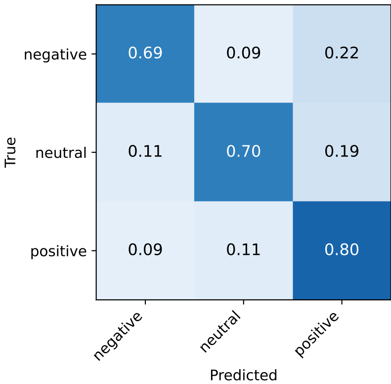
FinGPT-mt-Llama2-7B-LoRA
