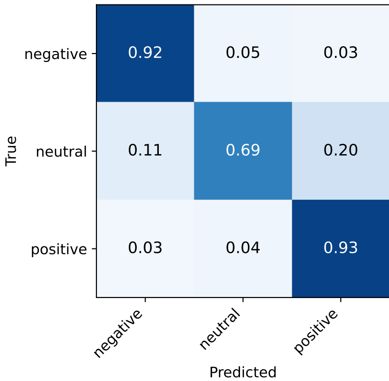
Finistral-7B-LoRA
