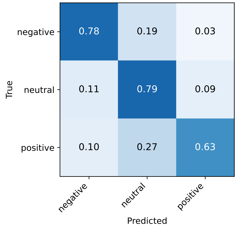
FinGPT-Llama-3-8B-LoRA
