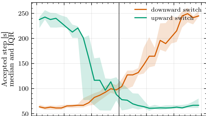
perilune start
