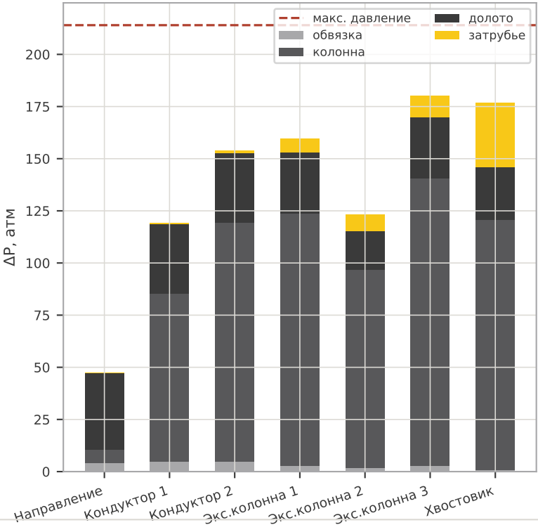
Баланс потерь давления
