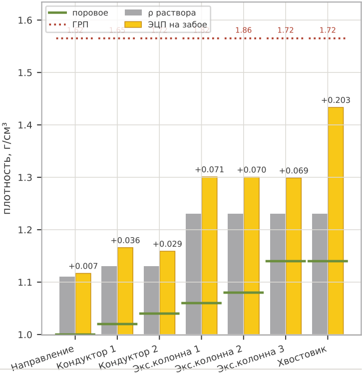
ЭЦП в окне бурения
