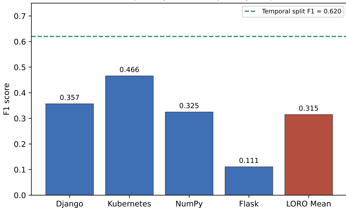
Leave-One-Repository-Out F1 vs. primary temporal F1
