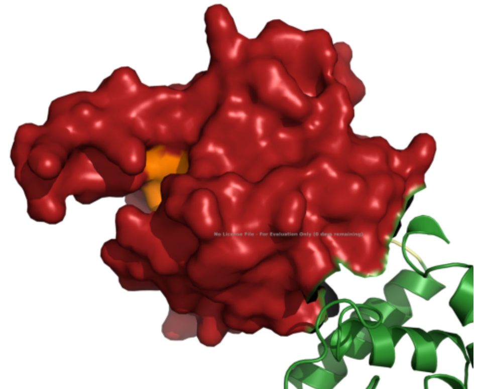
D — Catalytic groove
