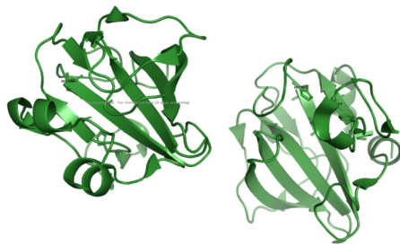
Lysostaphin (PDB 4QPB)
