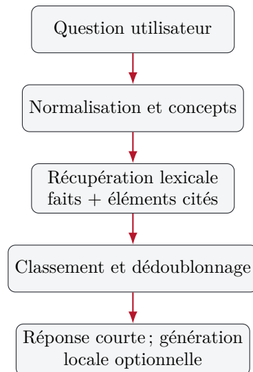
FIGURE 5.5 – Chaîne d’Ask Tender, sans embeddings ni index vectoriel.
