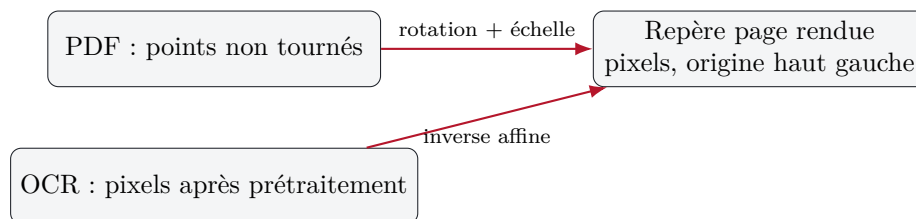
FIGURE 4.3 – Normalisation des boîtes natives et OCR vers le même espace d’affichage.
