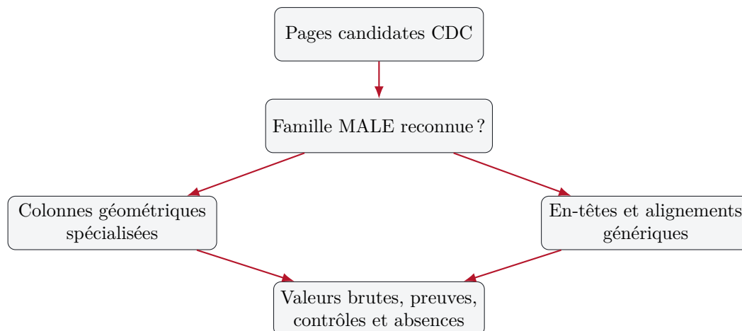
FIGURE 5.3 – Extraction BOQ spécialisée ou générique, suivie de contrôles explicites.
