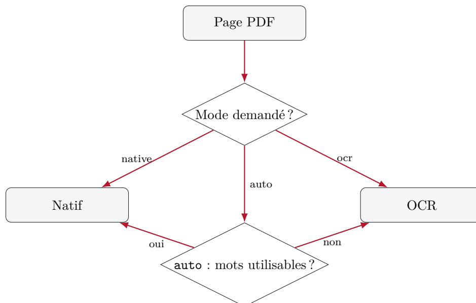
FIGURE 4.2 – Choix explicite du chemin pour une page ; le mode hybride garde les deux sources.
