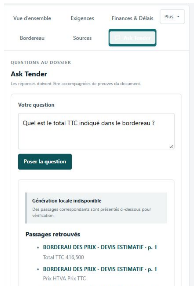
FIGURE 5.6 – Vue réelle d’Ask Tender sur une fixture BOQ synthétique : passages cités et indisponibilité explicite de la génération locale.
