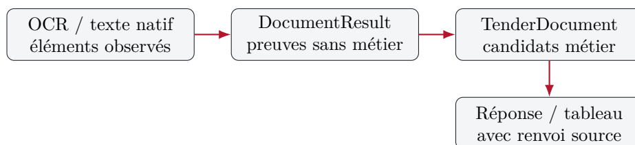
FIGURE 3.1 – Frontière entre reconnaissance, preuve normalisée et interprétation métier.
