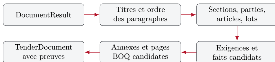
FIGURE 5.1 – Pipeline de l'analyse CDC à partir des éléments de preuve.
