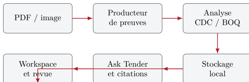
FIGURE 2.1 – Chaîne d'analyse et de restitution attestée par les modules du dépôt.
