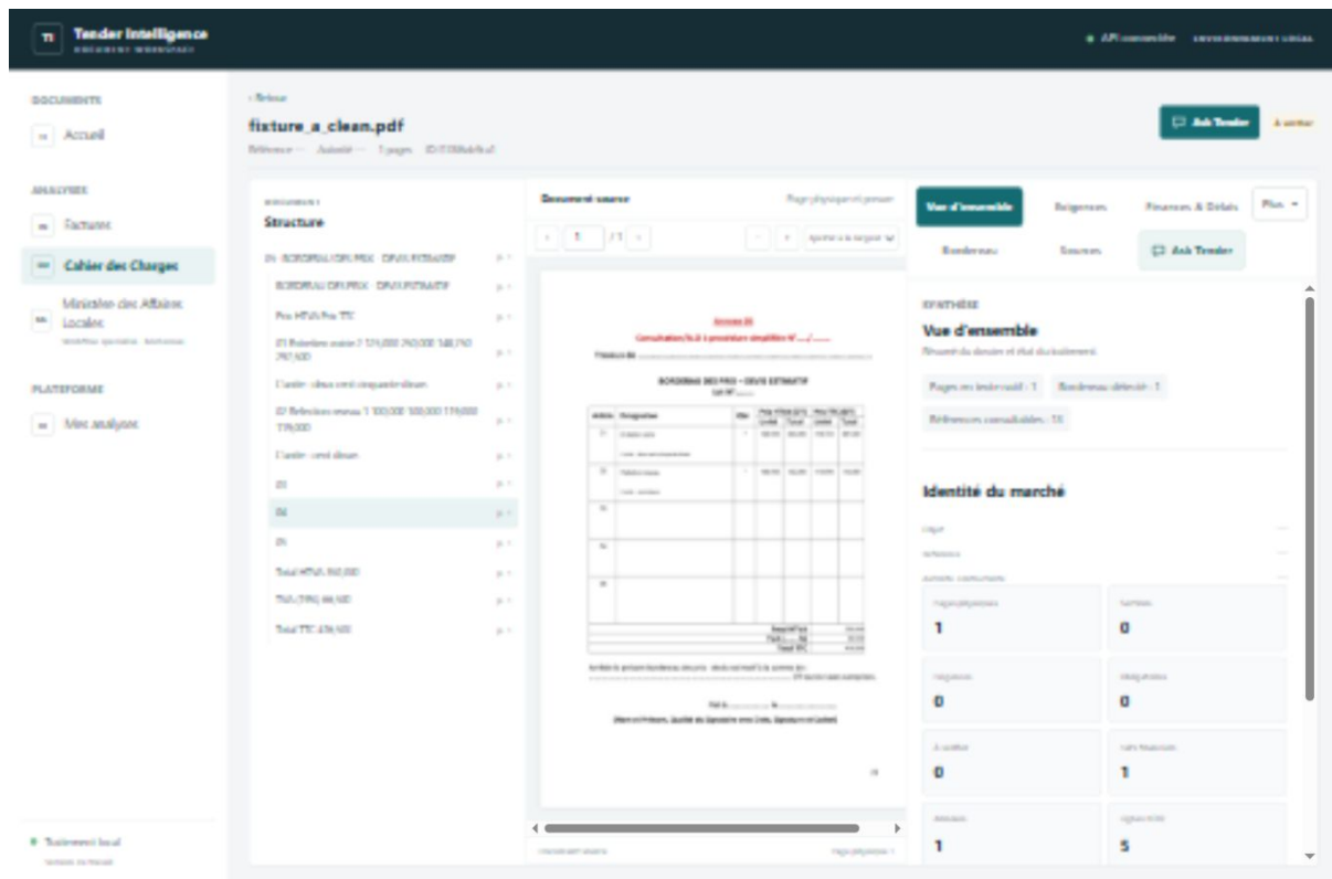
FIGURE 5.7 – Workspace exécuté localement avec la fixture BOQ synthétique : structure à gauche, document source au centre et analyse à droite.
