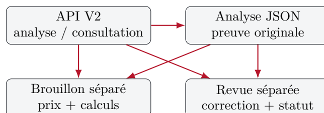
FIGURE 5.8 – Persistance locale : l'analyse source, la revue et le chiffrage sont des états distincts.
