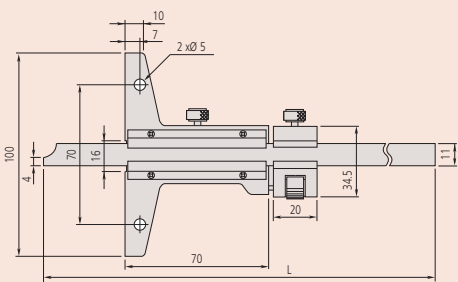
Capacité : 0-150 mm, 0-200 mm, 0-300 mm
