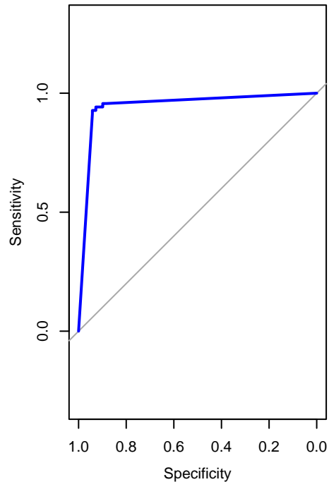
ANN (AUC = 0.946 )
