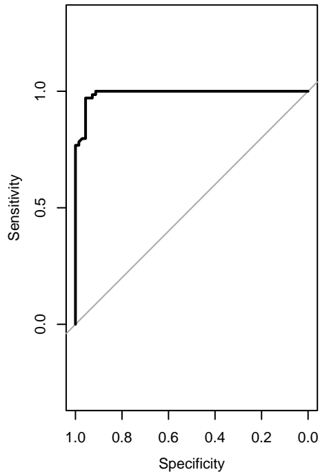
RF (AUC = 0.99 )
