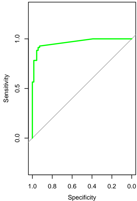
SVM (AUC = 0.965 )
