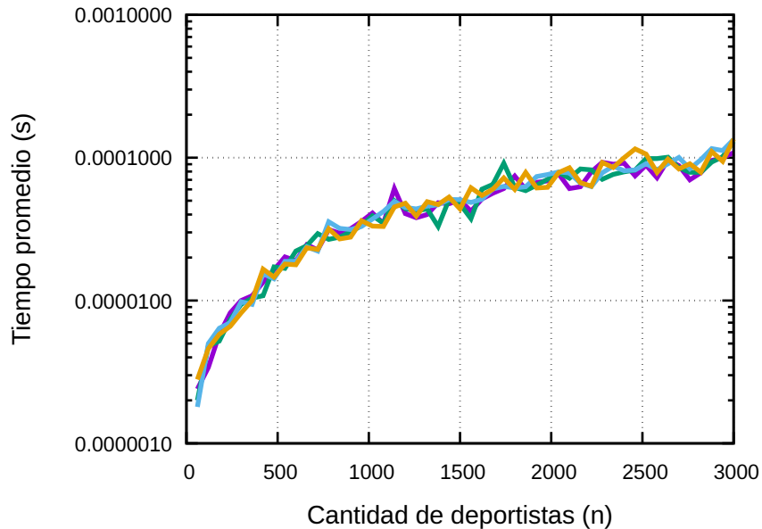
Quick Select benchmark - caso promedio
