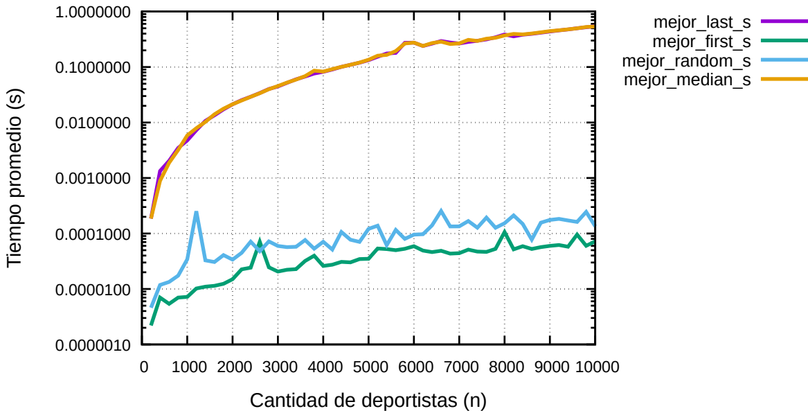
Quick Select benchmark - mejor caso
