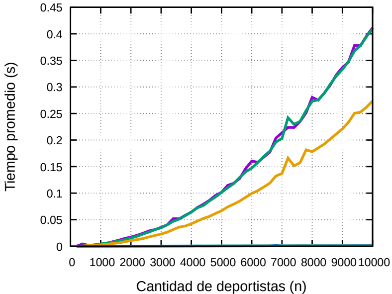
Sort benchmark - peor caso
