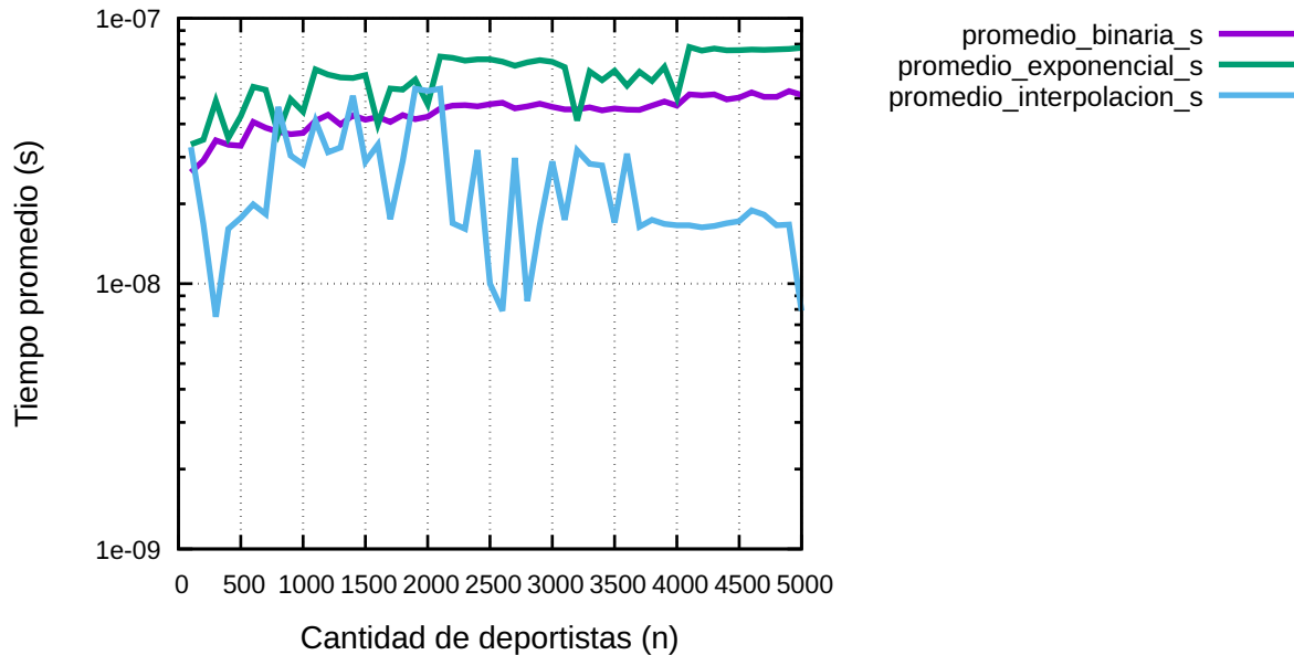
Search benchmark - caso promedio
