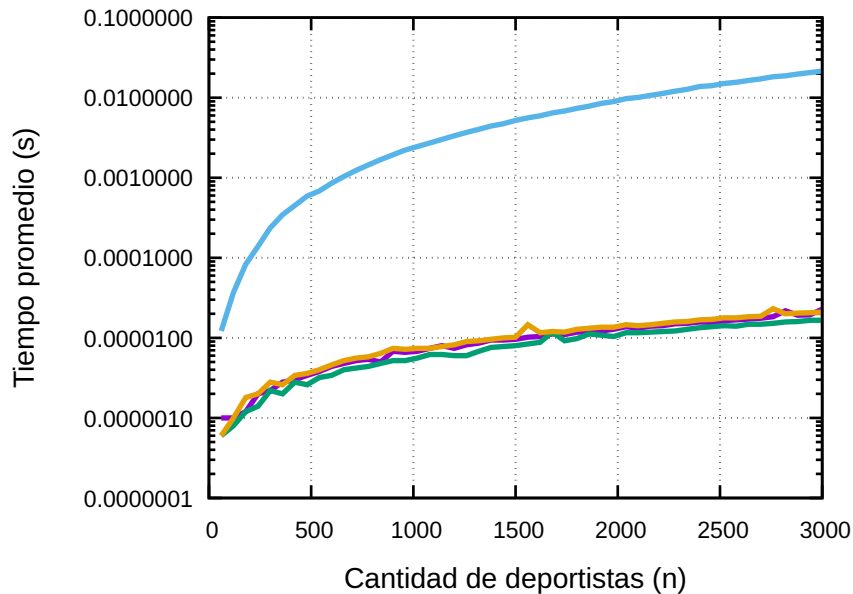
Sort benchmark - mejor caso
