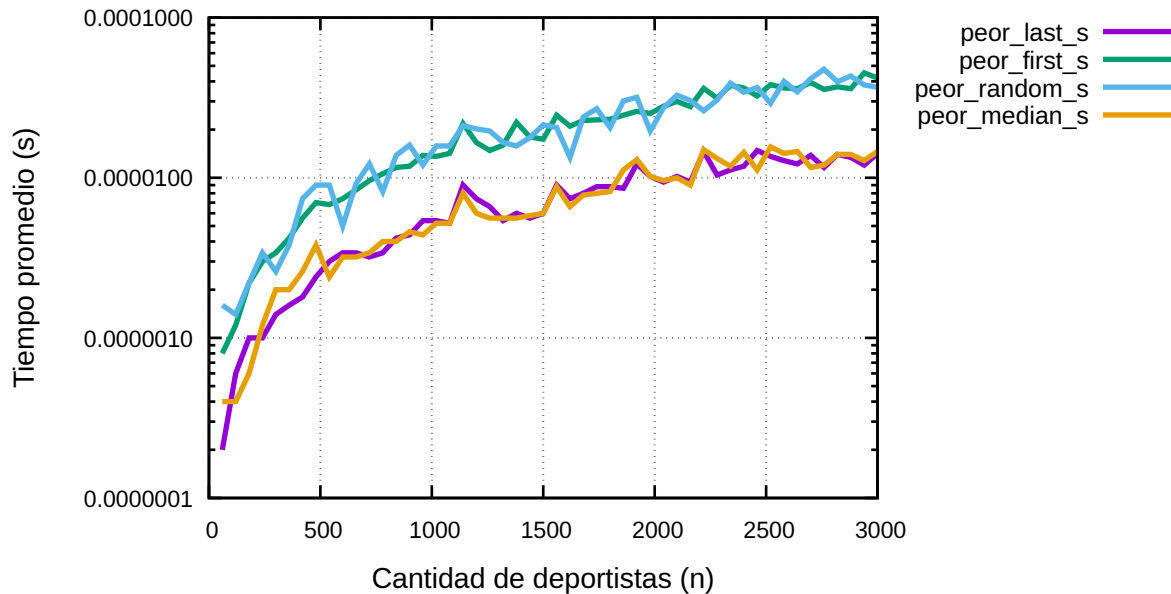
Quick Select benchmark - peor caso
