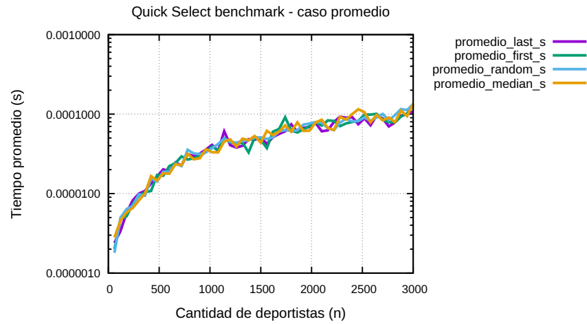
Figura 4.7: Benchmark de Quick Select en caso promedio.
