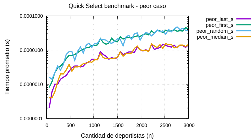
Figura 4.8: Benchmark de Quick Select en peor caso.
