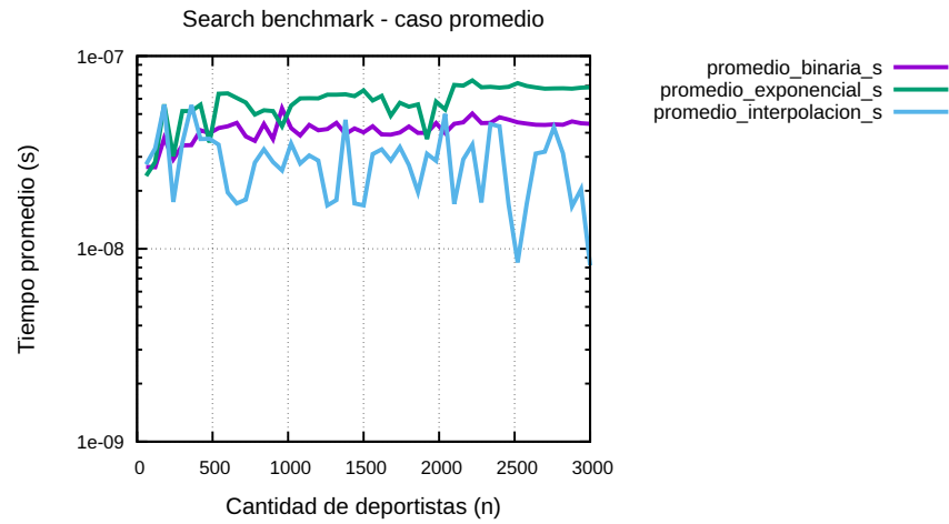
Figura 4.5: Benchmark de algoritmos de búsqueda en caso promedio.
