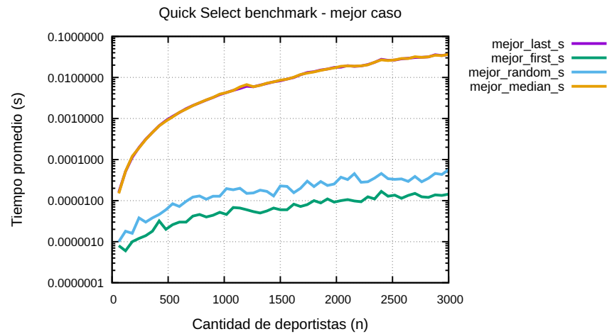
Figura 4.6: Benchmark de Quick Select en mejor caso.
