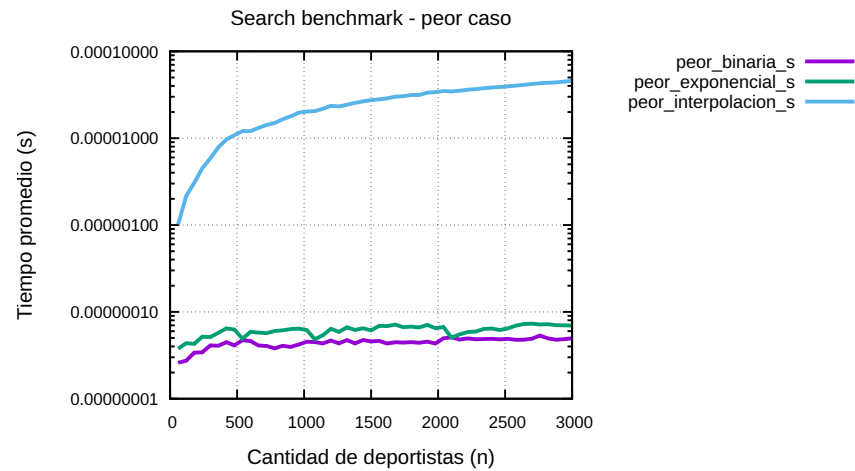
Figura 4.4: Benchmark de algoritmos de búsqueda en peor caso.
