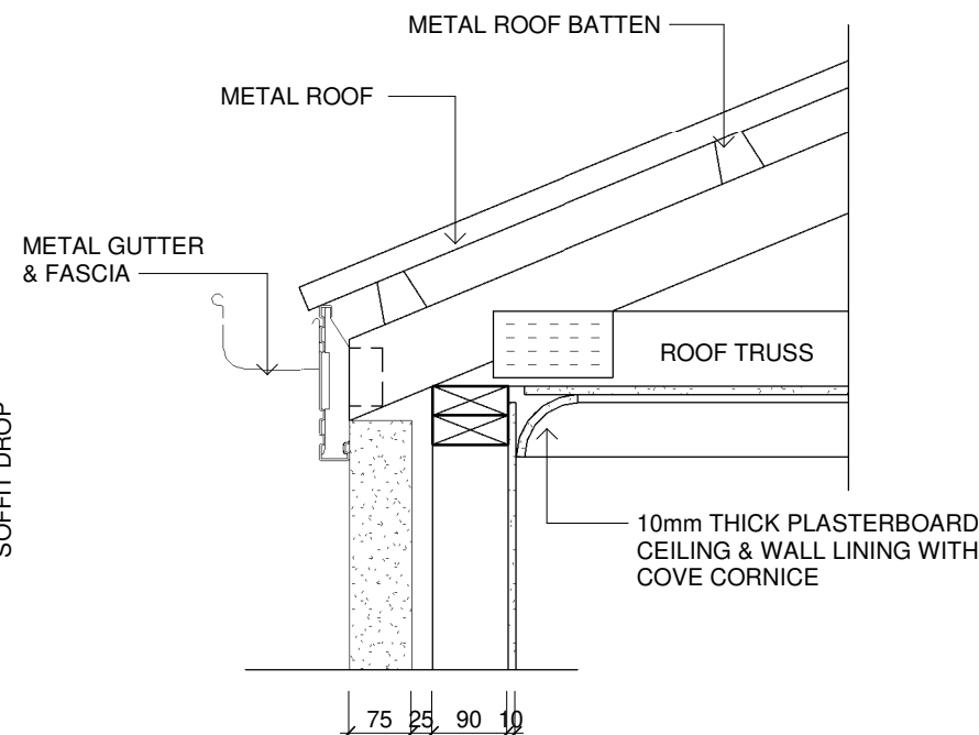
4 NO EAVE DETAIL 1 : 10
