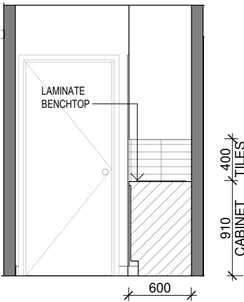
ELEVATION - LD
