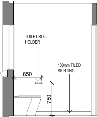
ELEVATION - WA
