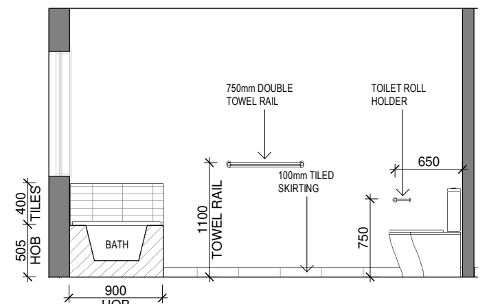
ELEVATION - ED
