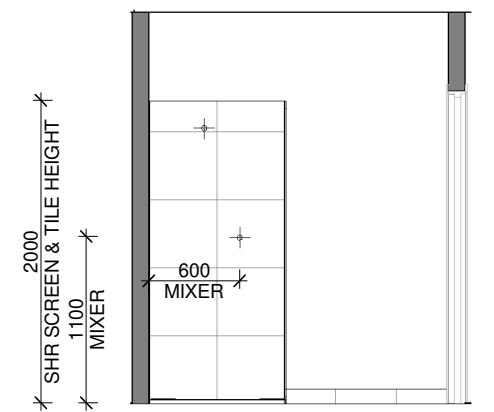
ELEVATION - BD
