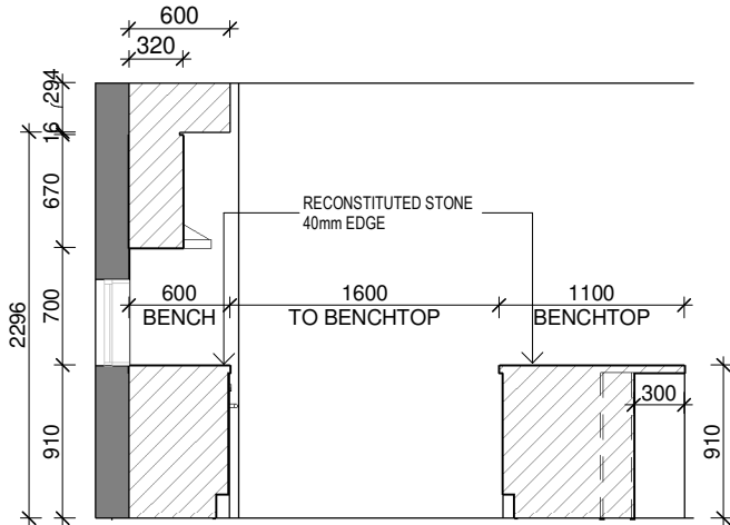
ELEVATION - KC
