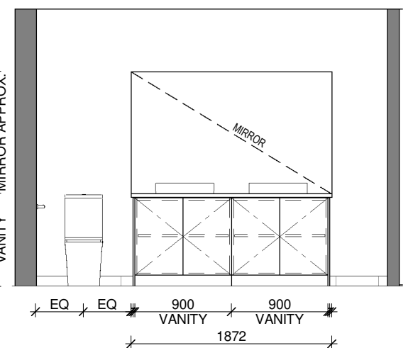
ELEVATION - EC
