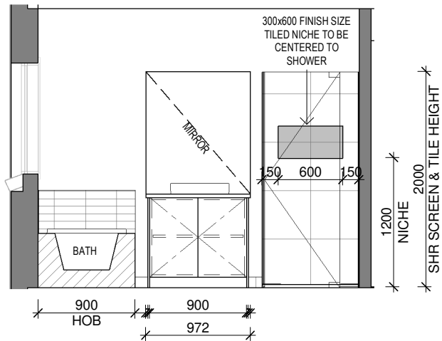
ELEVATION - BA
