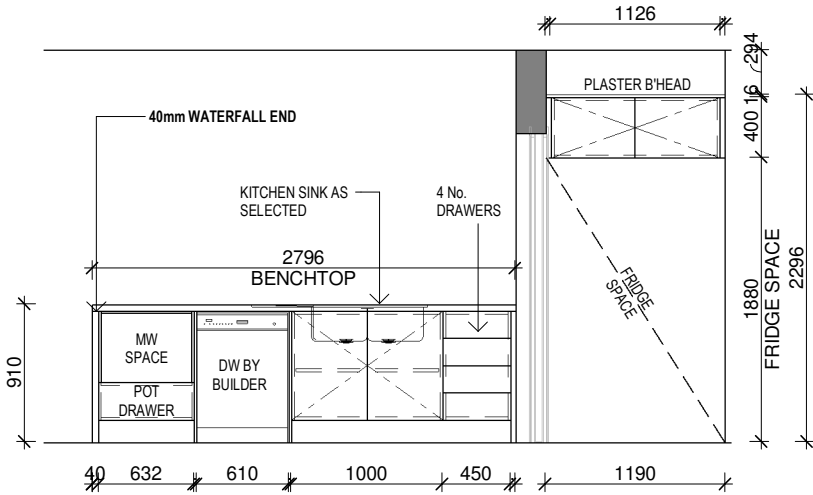
ELEVATION - KB
