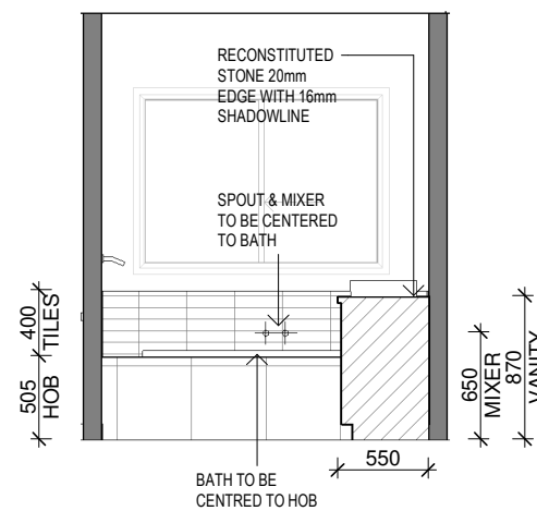
ELEVATION - BB
